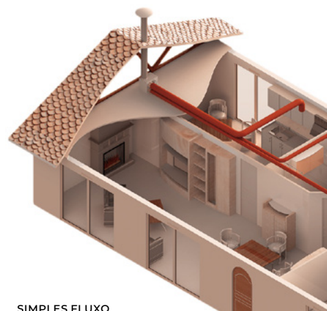
SIMPLES FLUXO
