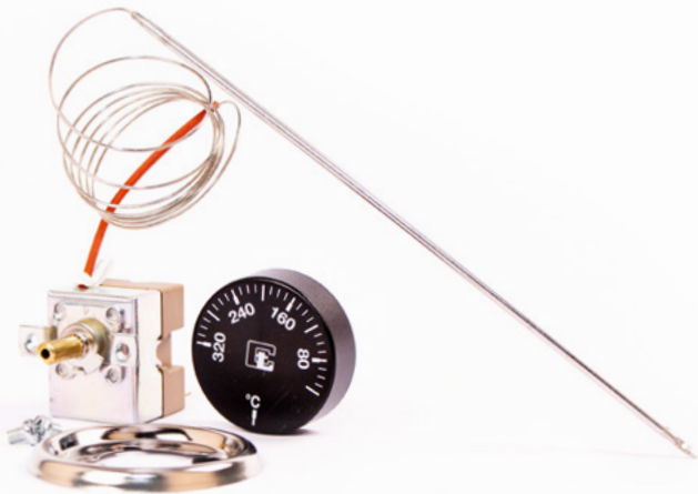
TERMOSTATO DE Sonda TVE3-50-320
